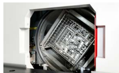
Un nettoyage ciblé par balancement et rotation du support de pièces
